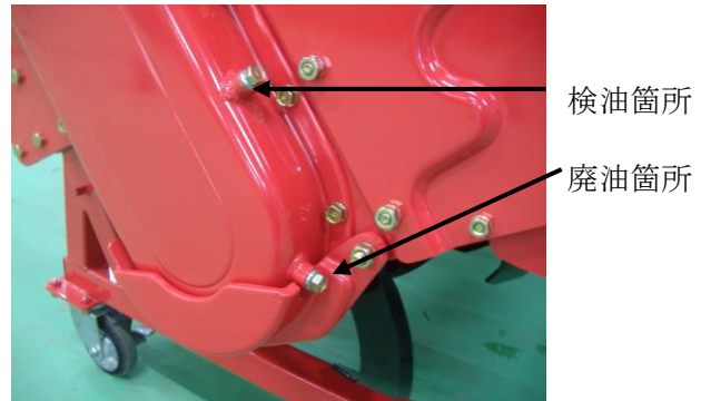
ケース下（ローター側）
